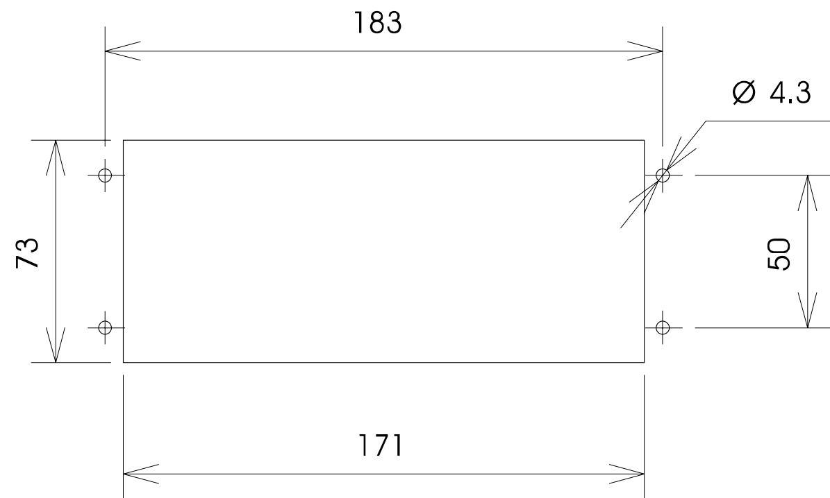
Montageöffnung / Mounting Opening
