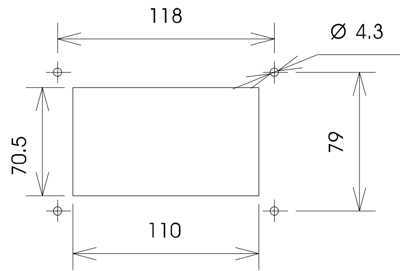
Montageöffnung / Mounting Opening
